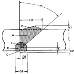
(3) 베벨형 판이음용접
