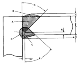
(6) 베벨형 모서리이음용접
