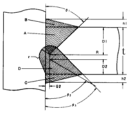
(9) K형 T이음용접
