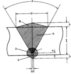
(4) V형 판이음용접
