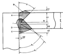
(7) K형 모서리이음용접
