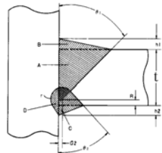
(8) 베벨형 T이음용접
